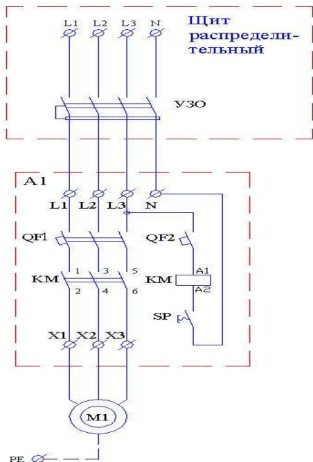
Эл.схема 1
