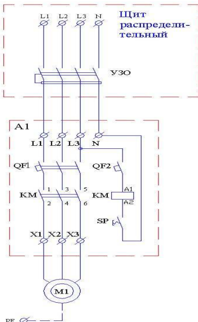
Эл.схема 2
