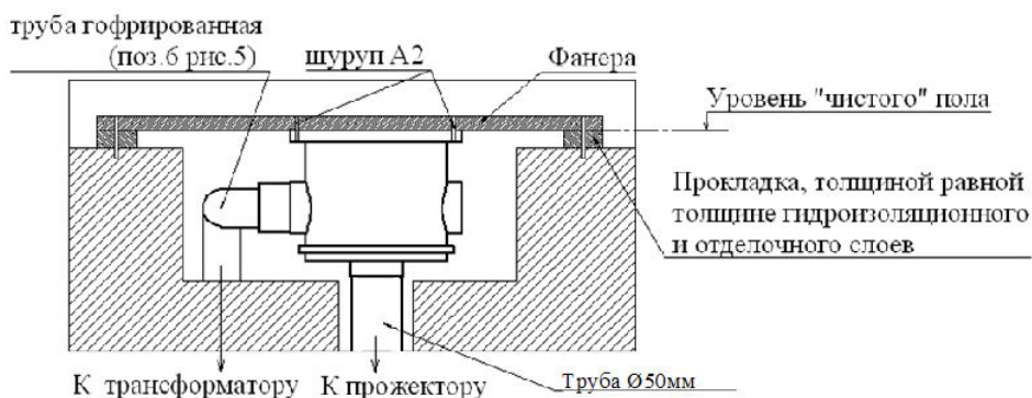
Закладной узел
