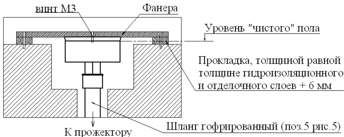
Закладной узел
