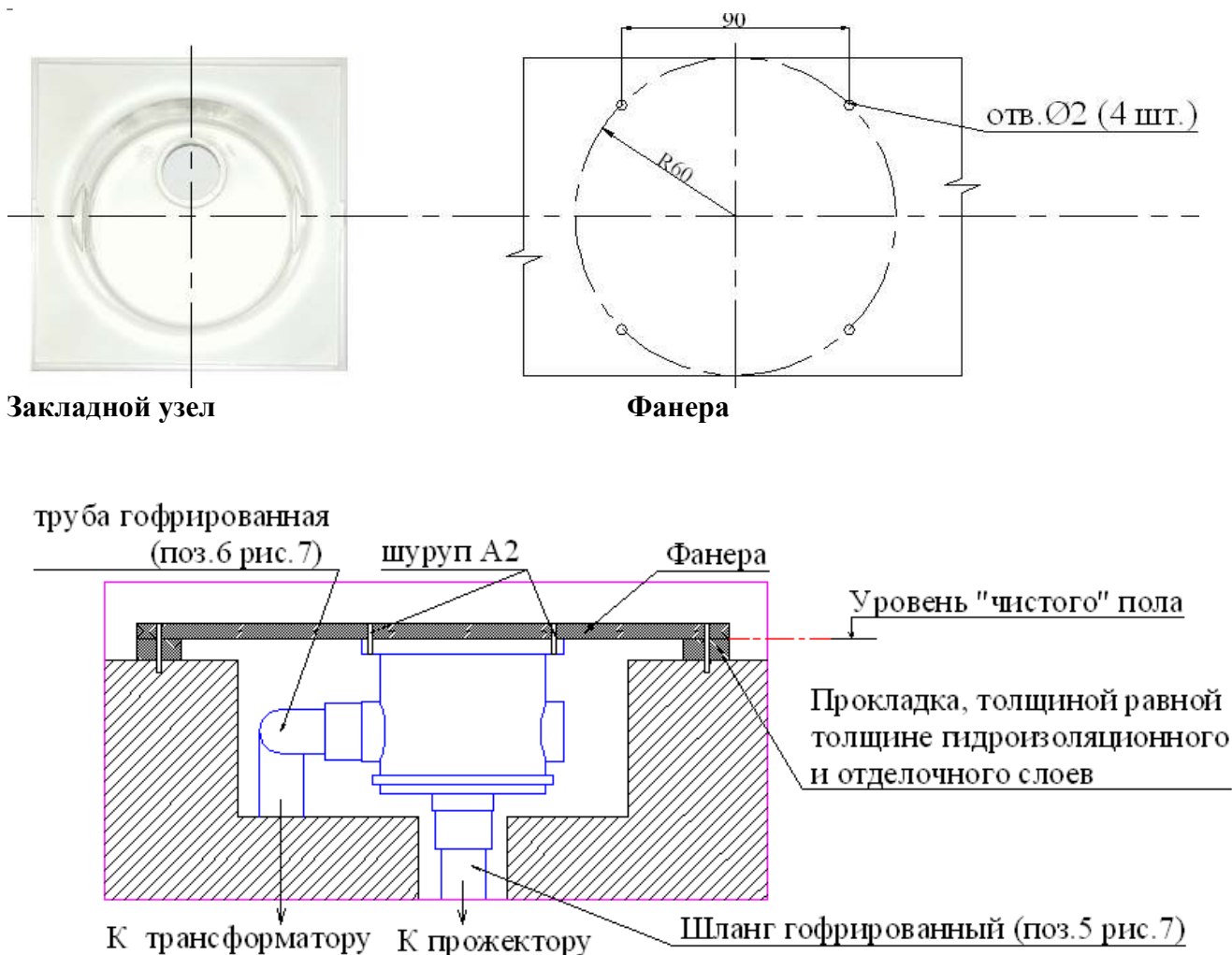
Рисунок 12 Установка короба распаячного Kripsol CX.C
