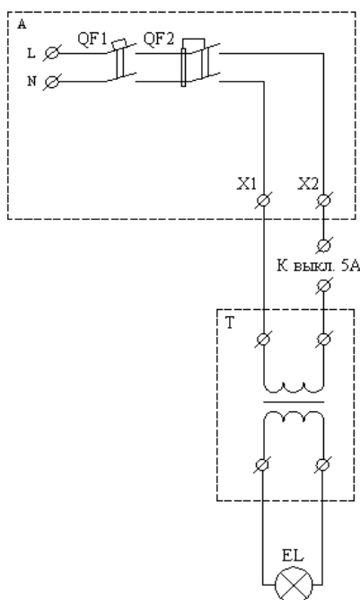
Электрическая схема 1
