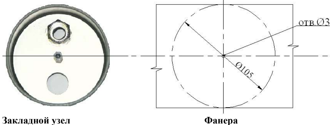
Рисунок 13 Установка короба распаячного из нерж. стали Pahlen (12310)
