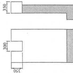
Ниша для регулятора уровня воды Kripsol RGPC
