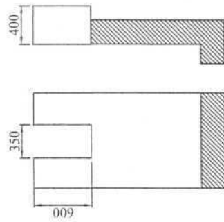
Ниша для скиммера Kripsol SKSL
