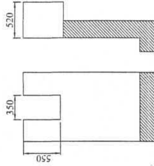
Ниша для форсунки противотока Kripsol HidroJet
