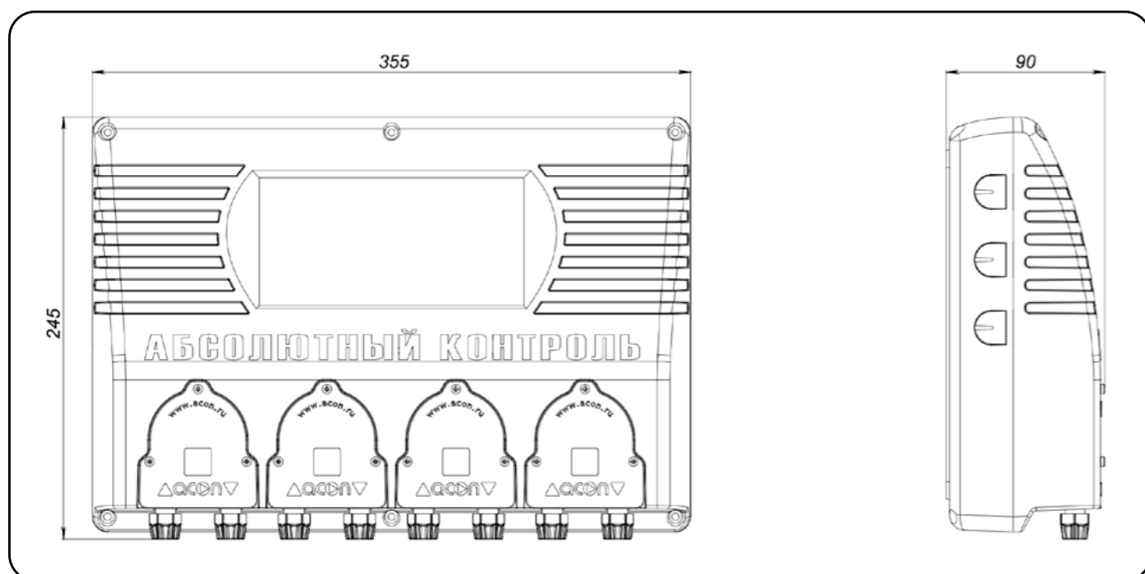
Рис.1 - Общие размеры Установки
