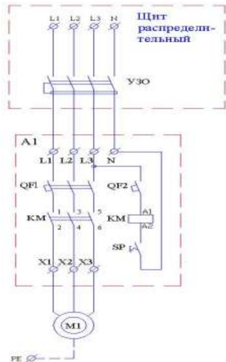
Эл.схема 1
